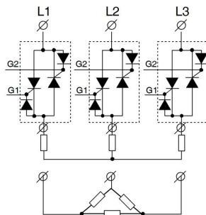
K9 三相三线全控功率模 块星型、三角形接线图 （单相可控硅反并联）
