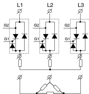
K9 三相三线半控功率模 块星型、三角形接线图 （单向可控硅+二极管）
