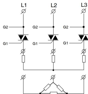
K9 三相三线星型、 三角形接线图（双向 可控硅）
